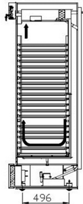
SECTION A-A
