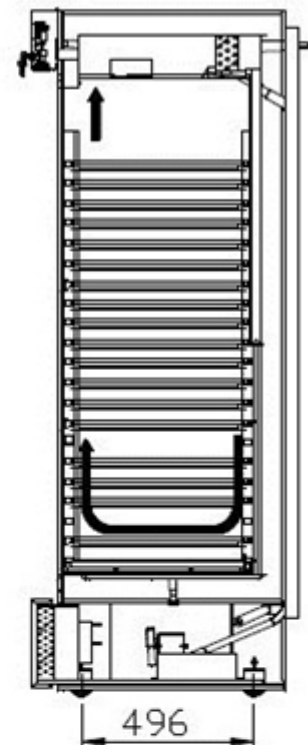
SECTION A-A
