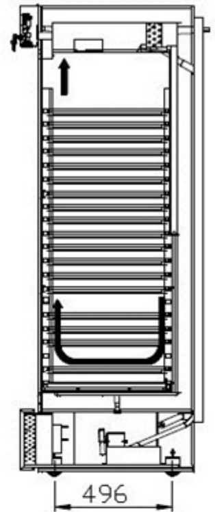
SECTION A-A
