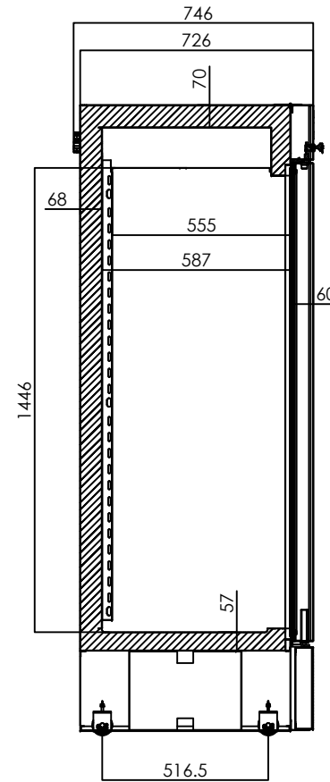
SECTION A-A
