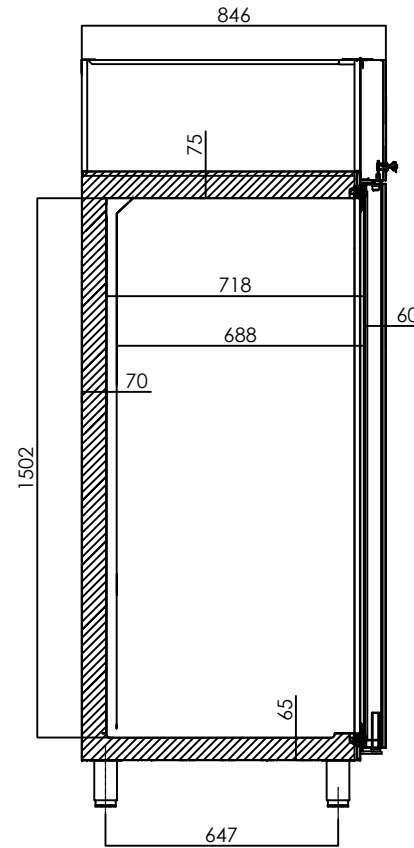
SECTION A-A
