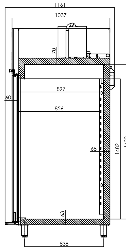
SECTION A-A
