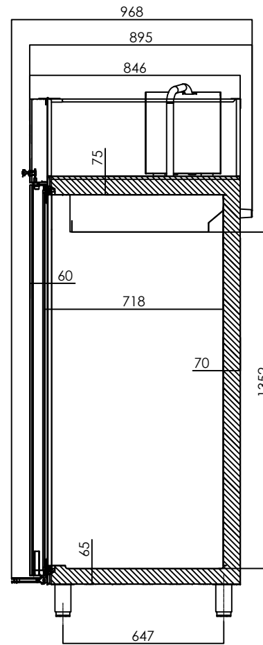
SECTION A-A
