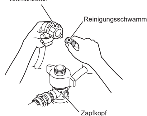
Schnellverbinder für Bierschlauch
